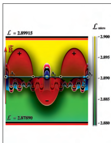
Рис.3.3.17. Переменное магнитное поле B представляет собой пери-
