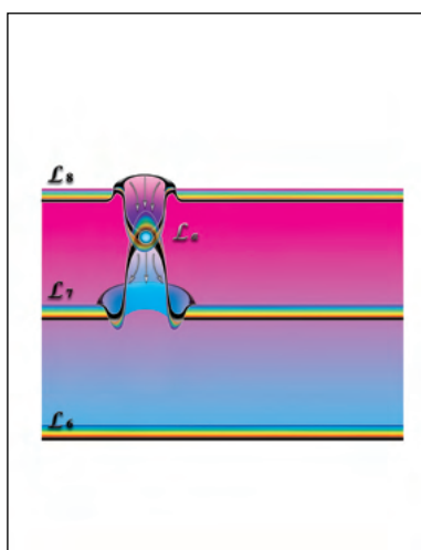
Рис.2.4.1. Возникновение звезды, при смыкании пространства-вселенной нашей мерности с пространством-вселенной большей мерности.
