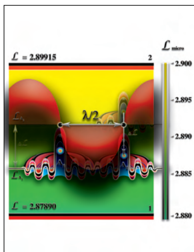
Рис.3.3.11. Возможность для атомов, имеющих разные уровни соб-
