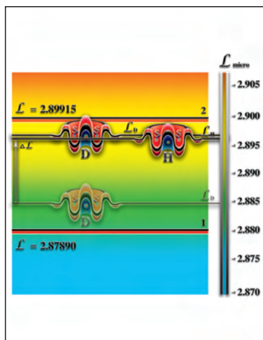
Рис. 3.3.8. Радиоактивный изотоп водорода — дейтерий D — вне за-
