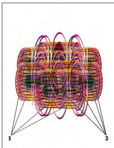
Рис.2.3.9. Суперпространство четвёртого порядка. Возмущение мер-
