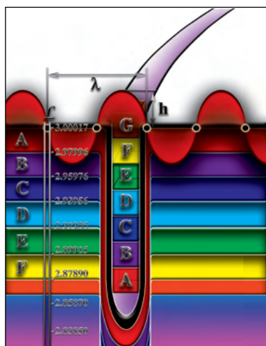
Рис. 3.2.10. После прохода фронта волны через данную точку про-
