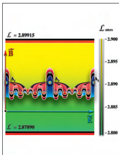
Рис.3.3.14. Кристаллическая решётка любого твёрдого вещества не-
