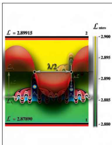
Рис.3.2.11. При образования ядра атома, возникают возмущения
