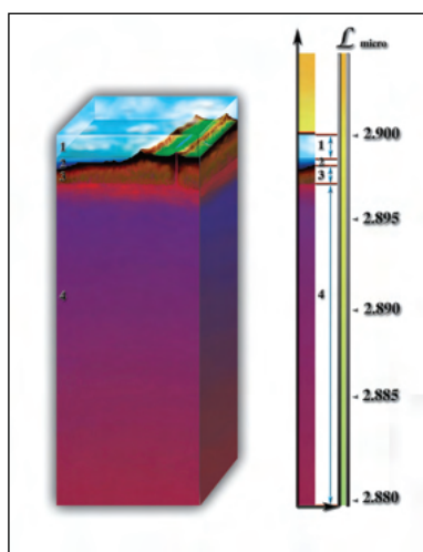
Рис. 3.3.9. Каждая молекула или атом имеют свой диапазон мерно-
