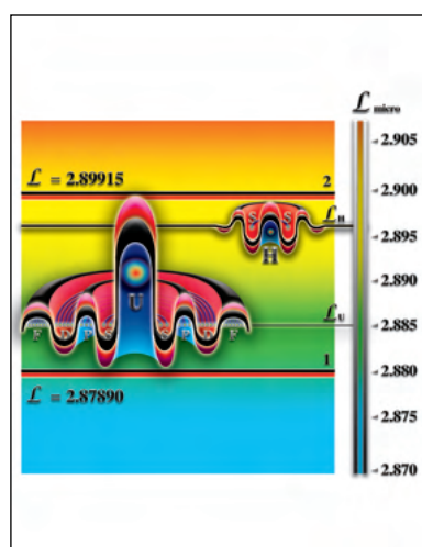
Рис.3.3.5. Сопоставление степени влияния на окружающий микро-
