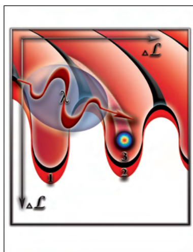
Рис.3.2.14. «Смерть» электрона может произойти на одной орбите,
